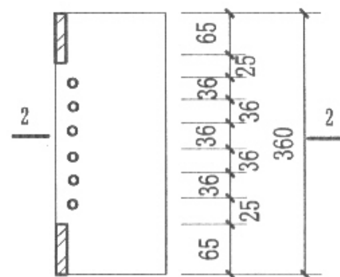
铸铁篦子
