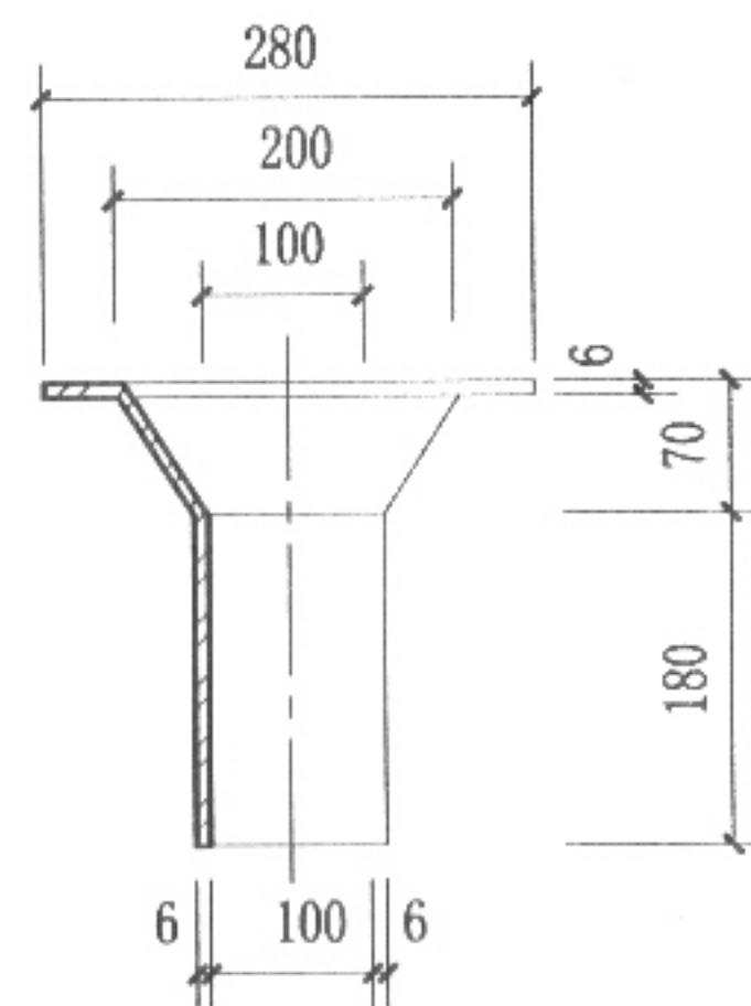
(E) 铸铁雨水口底座
