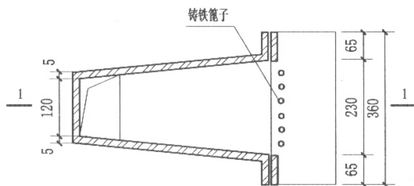
1 铸铁雨水口
