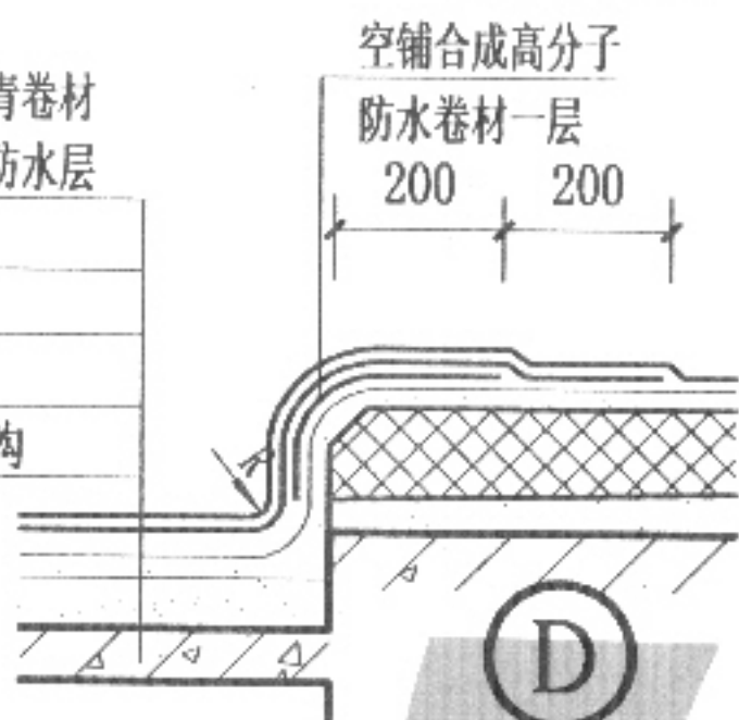
(卷材, 涂膜屋面)
