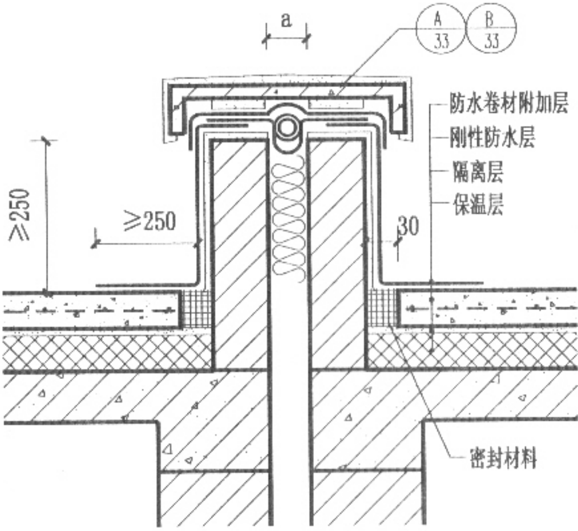
② 有保温屋面变形缝
