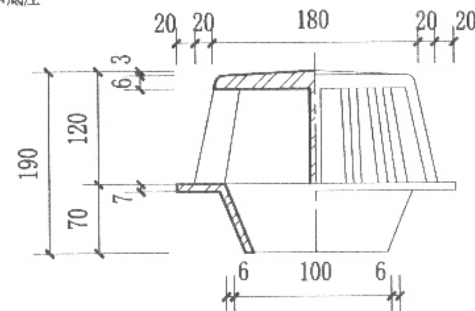
(F) 铸铁雨水口上口
