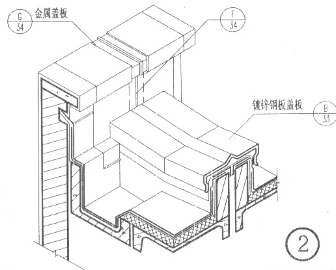
女儿墙屋面变形缝 (一)
